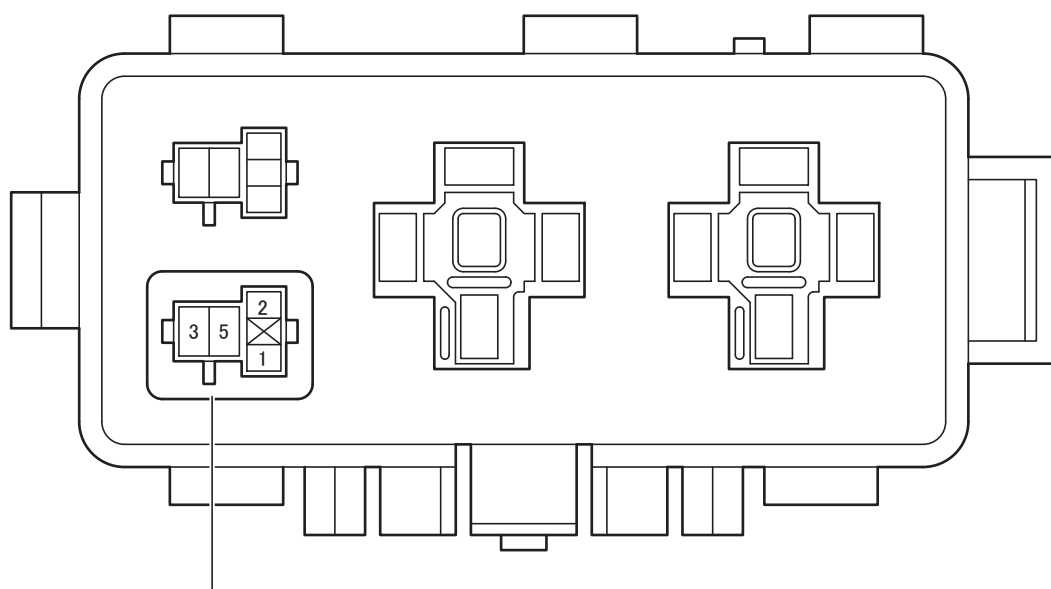
DEICERリレー
